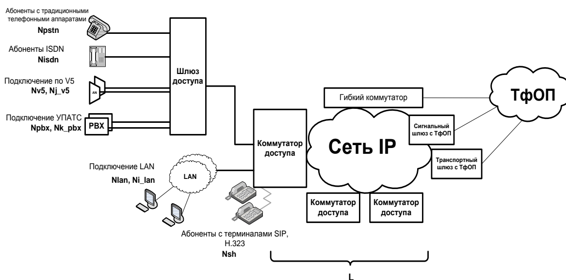
ис. 10. Параметры оборудования сети доступа
