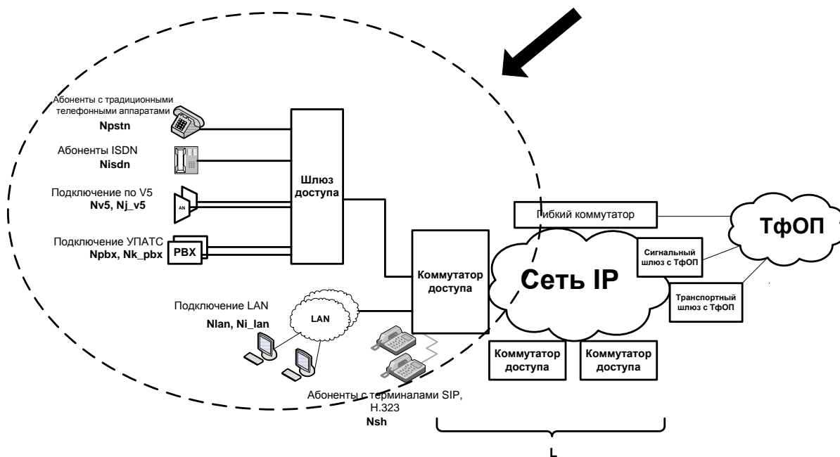
ис. 7. Шлюз доступа в сети NGN
